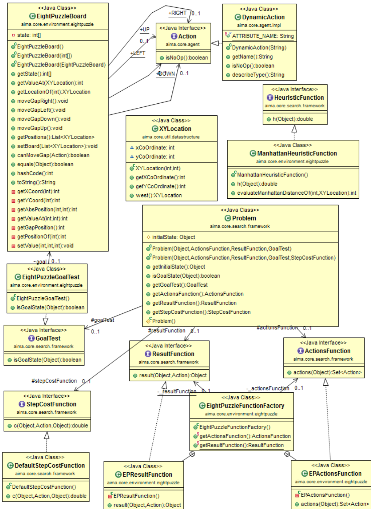
Figura 1: Diagrama de clases para la implementación del espacio de estados del N-puzzle en el framework aimajava.
