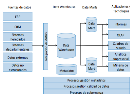
Figura 1: Arquitectura de un sistema BI.
