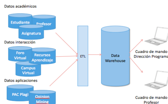
Figura 3: Arquitectura BI para docentes.
