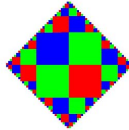
Figura 7. Solución del problema de coloreado
