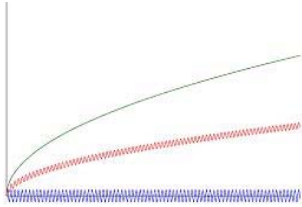
Figura 1. Representación de dos funciones y su media
