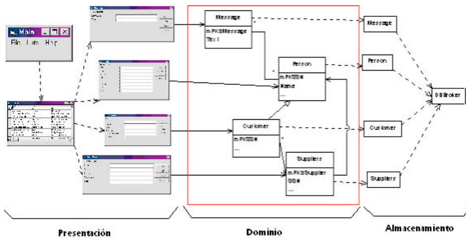
Figura 5. Fragmento de la estructura de una de las aplicaciones generadas.
